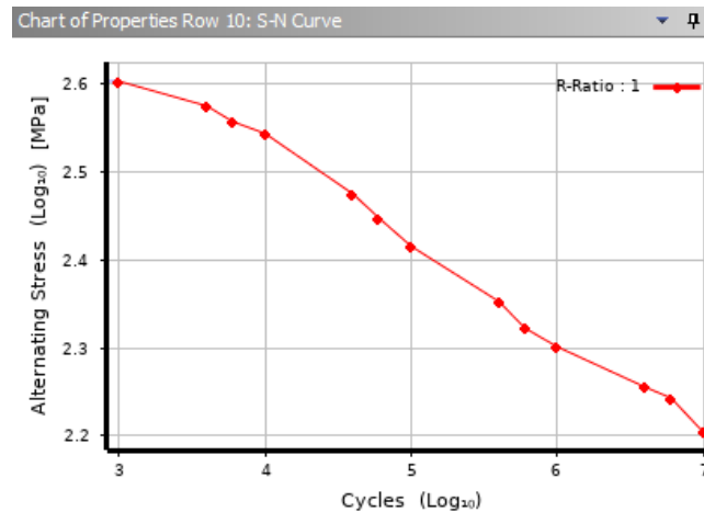
Figura 8. Curva S-N del acero A-36
