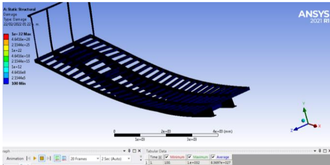
Figura 23. Daño a fatiga de la estructura
