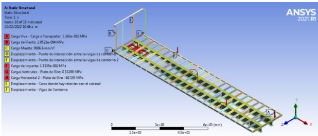
Figura 9. Cargas y soportes aplicados en la plataforma
