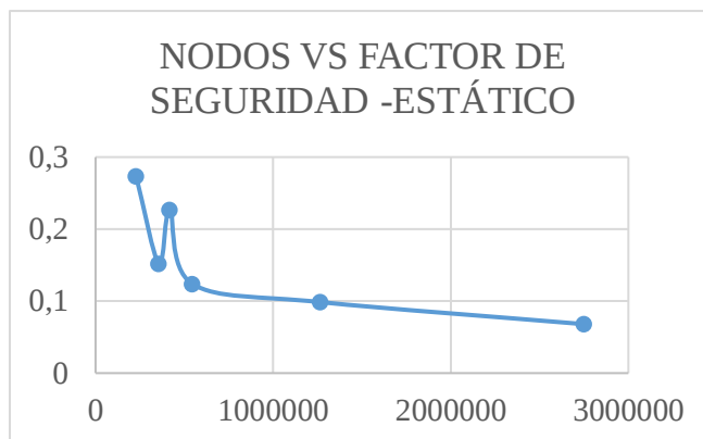
Figura 14. Gráfica de convergencia en Factor de seguridad
