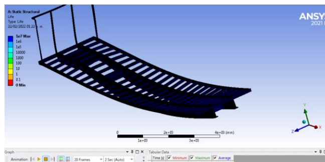
Figura 22. Vida a fatiga de la estructura
