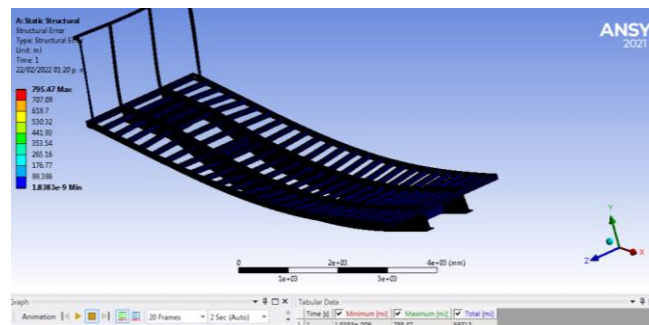
Figura 20. Error estructural
