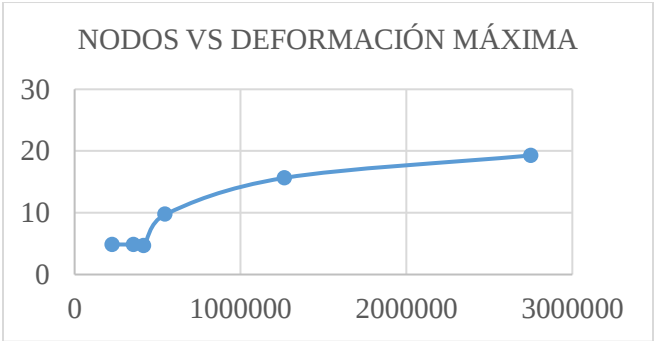
Figura 12. Gráfica de convergencia en deformación total
