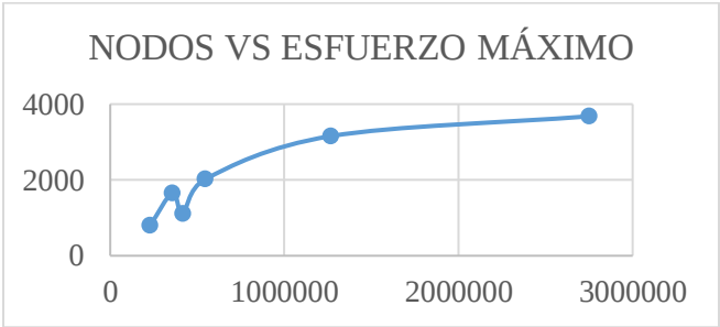
Figura 13. Grafica de convergencia en esfuerzo máximo
