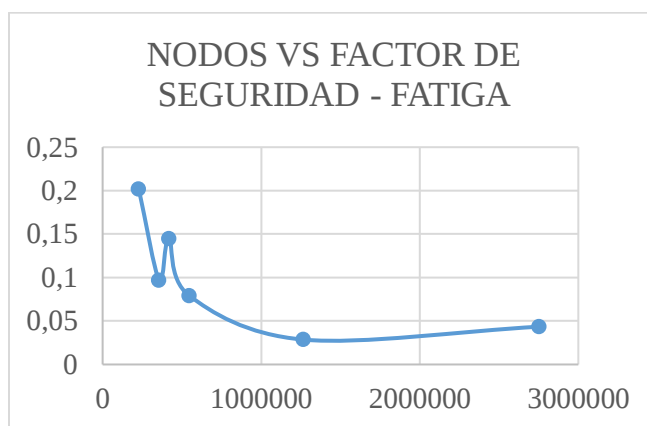
Figura 15. Gráfica de convergencia en Fatiga
