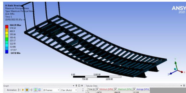
Figura 19. Esfuerzo principal máximo
