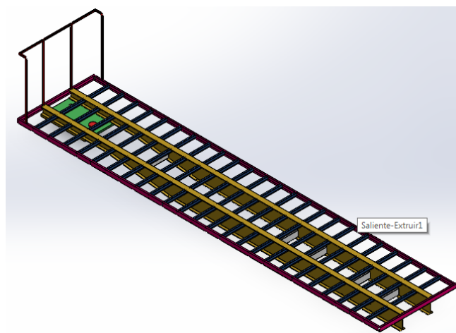
Figura 5. Asignación de perfiles a la plataforma de cama alta
