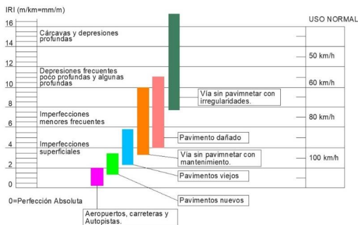
Figura 2. Escala de rugosidad
