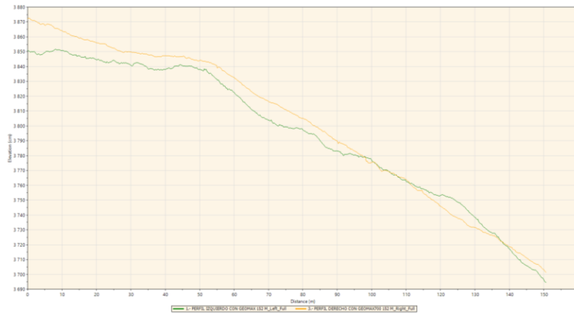
Figura 5. Perfil longitudinal con Nivel Electrónico de huella izquierda y derecha
