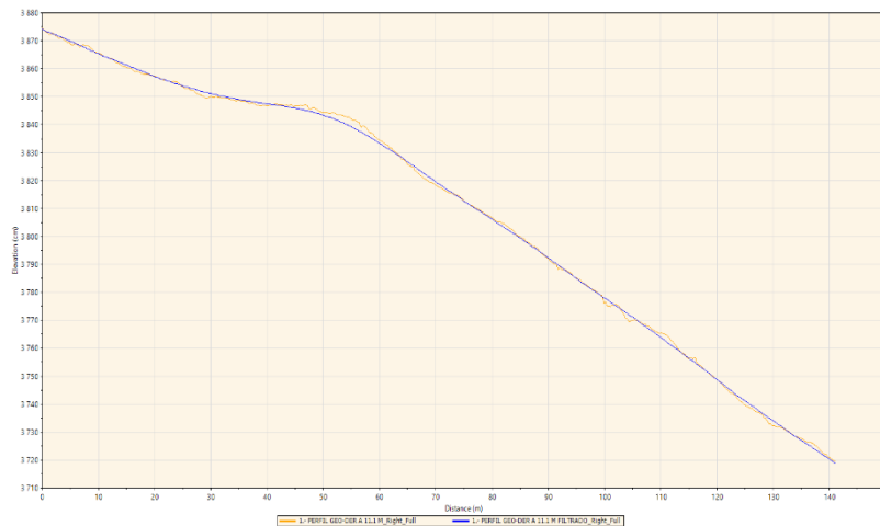
Figura 7. Ejemplo de Perfil filtrado Media Móvil base= 22.20 m.
