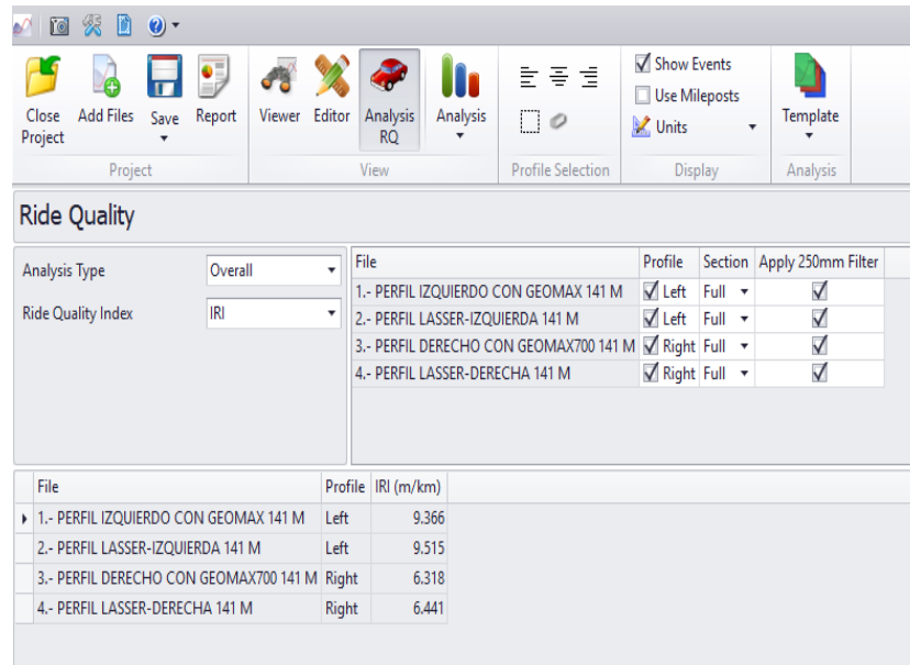
Figura 11. Resultados del IRI con ProVAL 3.61
