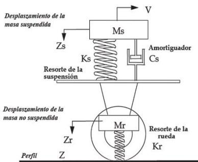
Figura 1. Modelo de cuarto de carro
