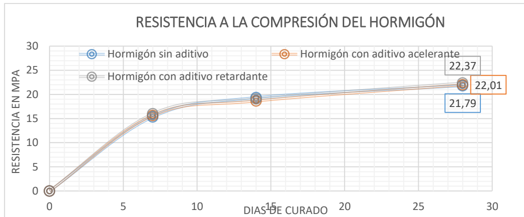
Figura 5 Resistencia a la compresión del hormigón agregados de Santo Domingo
