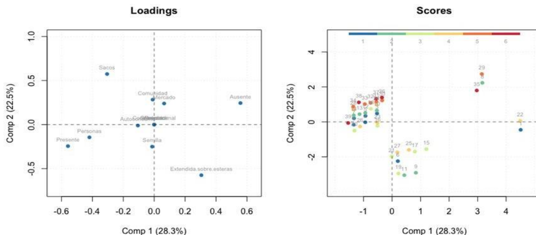
Figura 2. Análisis de componentes principales (PCA) que muestra los scores y las variables para el estudio de la diversidad de maíz. Los números 1 al 6 corresponden a las comunidades monitoreadas en este estudio.
